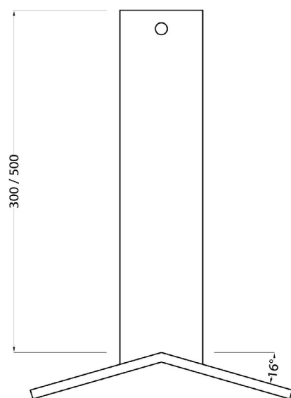
VISTA FRONTALE
